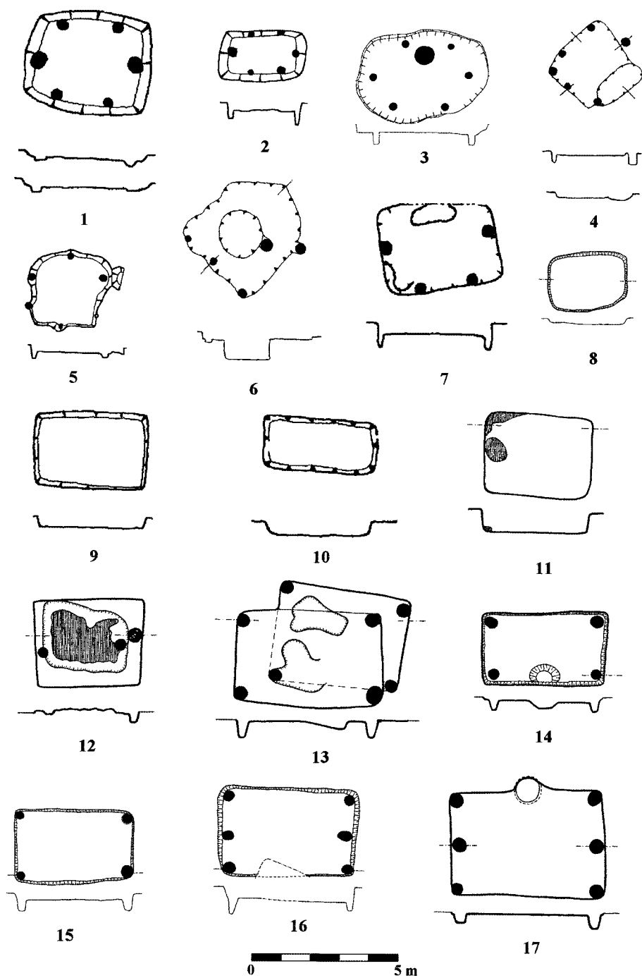
5. Půdorysy zahloubených germánských chat. 1–2,9 Mikulčice (podle Peškař 1961b), 3 Uherský Brod (podle Geisler–Kohoutek 2000), 4,6 Vlčnov-Dolní Němč, 5 Havříce (podle Geisler 1994), 7 Ostrožská Nová Ves (podle Galuška 1988), 8,11–17 Zlechov, 10 Drslavice (podle Pavelčík 1950).
