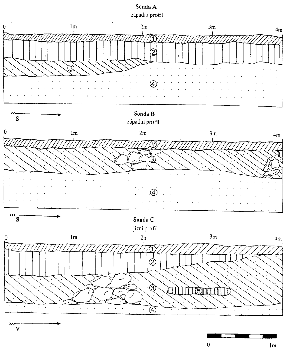
3. Profily sond A, B a C s následnou stratigrafií (vrstva 1 – vrstva humusu na povrchu lokality, vrstva 2 – stavební suť s úlomky cihel a dlaždic, vrstva 3 – černě zbarvená kulturní vrstva s pravěkými nálezy, vrstva 4 – jílovité podloží, vrstva 5 – mazaniceová kry).
